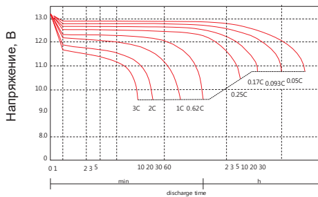
Напряжение разряда, в зависимости от времени
